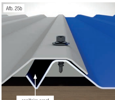
damwandprofiel 20/1100
